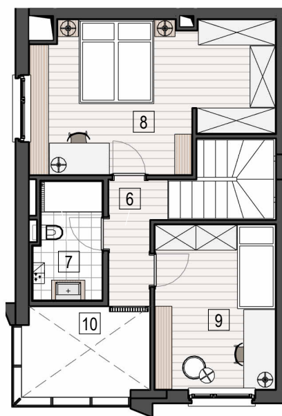
GORNJA ETAŽA
